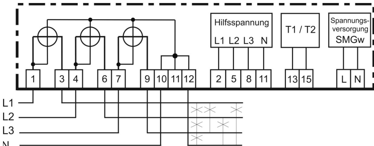
Abb. 5: Schaltbeispiel
